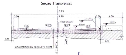
DETALHE - 01 SEM ESCALA
