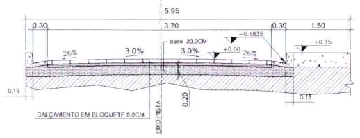
Seção Transversal
