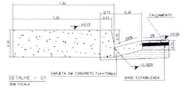
Seção Transversal
